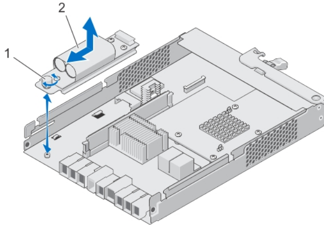
Figure 25. RAID 컨트롤러 모듈 백업 배터리 장치 분리 및 설치
